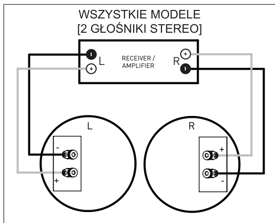
Rys. 5a Okablowanie dla wszystkich modeli z wyjątkiem H65-SM v.2, patrz poniżej.
