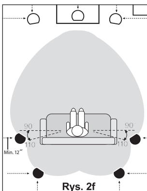
Rys. 2f 7.1 kolumny o bezpośrednim rozproszeniu dźwięku
